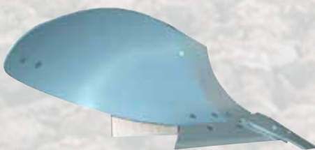
Corps UC pour un agressif en 14°.
