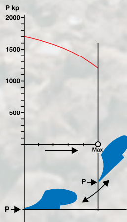
Sécurité hydraulique - dégagement vertical de 50cm.
