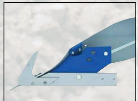
Coudre incorporé avancé améliore la qualité du labour en coupant le sol avant le retournement.
