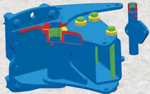
Tous les pivots du système Vari Flex sont équipés de bagues d'usures et de graisseurs.
