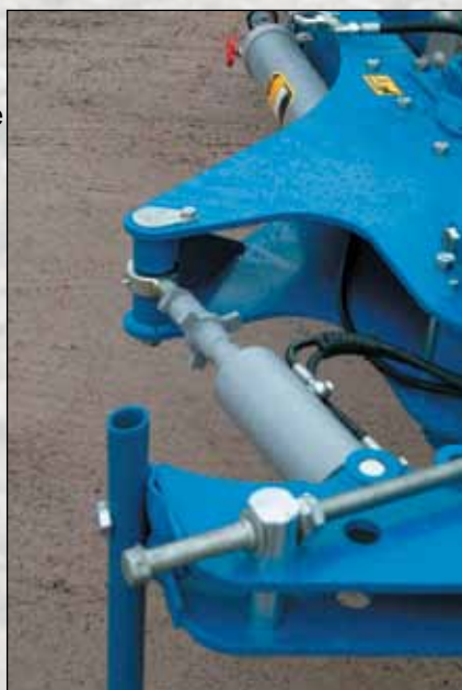
Le vérin the réalignement automatique recentre la charrue lors du retournement puis la remet dans la position prérégler.
