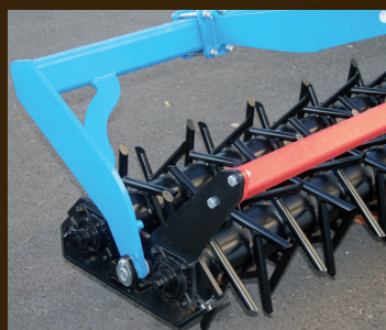
• Rouleau bipenta, double rotor Ø400 à dents Ø25
