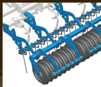
• Rouleau disque alvéolé Ø600 pas de 150 + peigne Ø16
