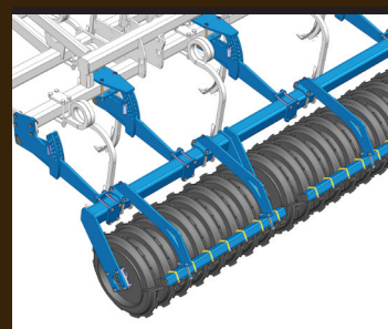
• Rouleau disque alvéolé Ø600 pas de 150
