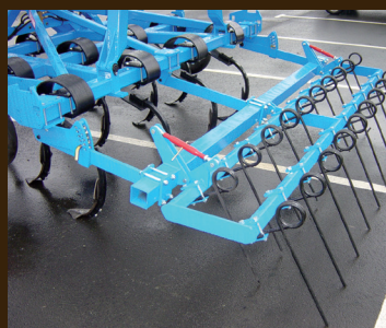
• Herse peignes escamotable, Ø16 sur 2 barres. Longueur utile 500 mm
