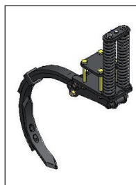
• Dent Chisel bilame 55x25 + 20. Dégagement 690 mm
